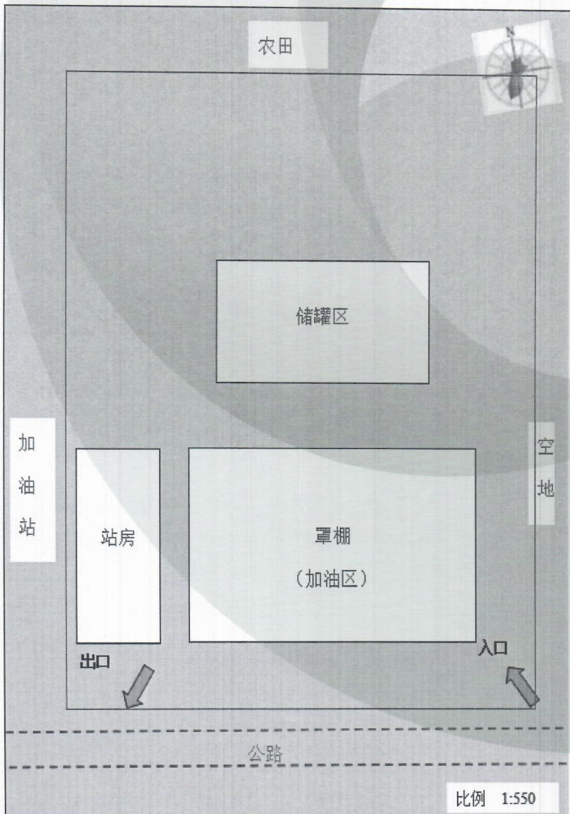
图 3-2 本项目平面布置图
