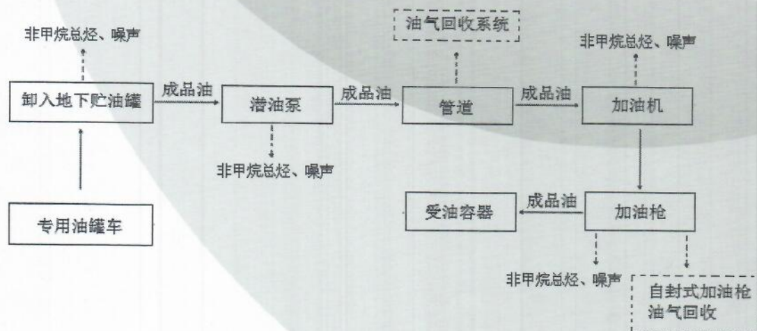
图 3-3 加油站工艺流程图
