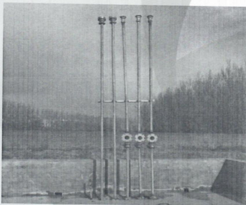
图 4-2 罐区通气管
