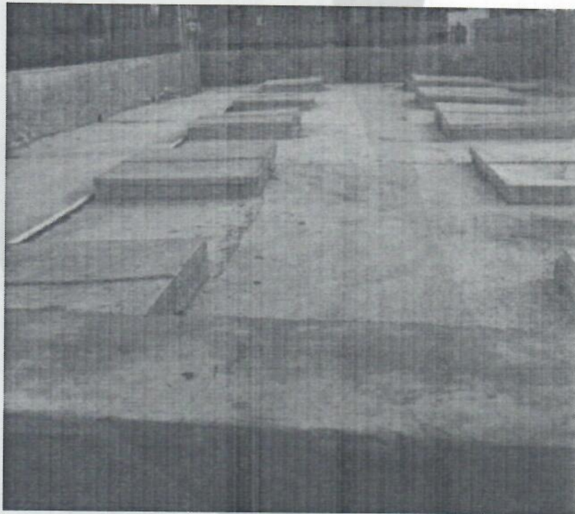
图 4-3 罐区围堰
